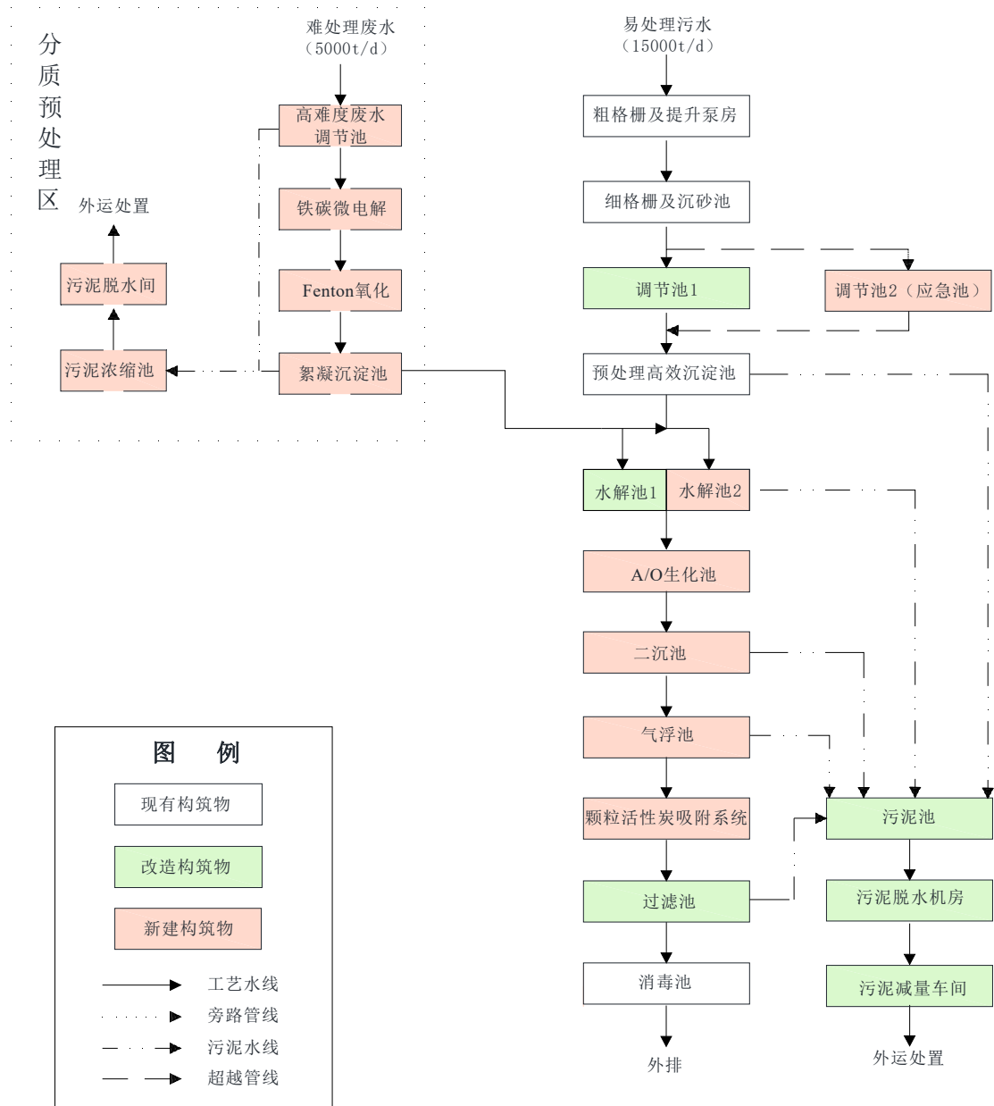
图7.1.3 淮安盐化新材料产业园区污水处理厂工艺流程示意图
