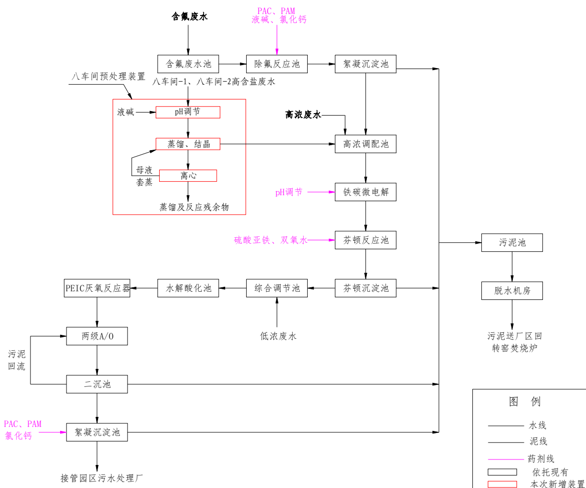
图7.1.2-1 扩建后，全厂废水处理工艺流程
