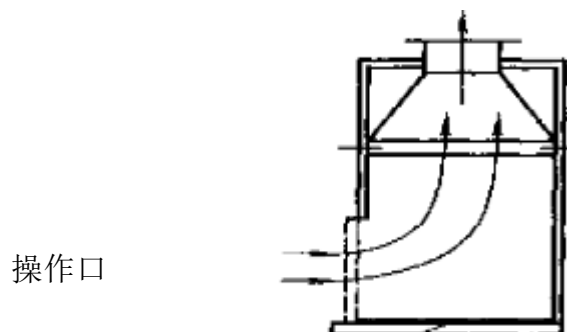
图7.2.1-1 拟建项目集气罩示意图
