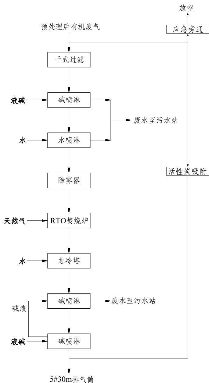
图7.2.1-4 RTO废气集中处理工艺
