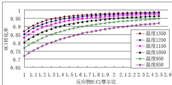
图4.4.1-1 各种温度工况下，反应物H/Cl比与HCl转化率的关系
