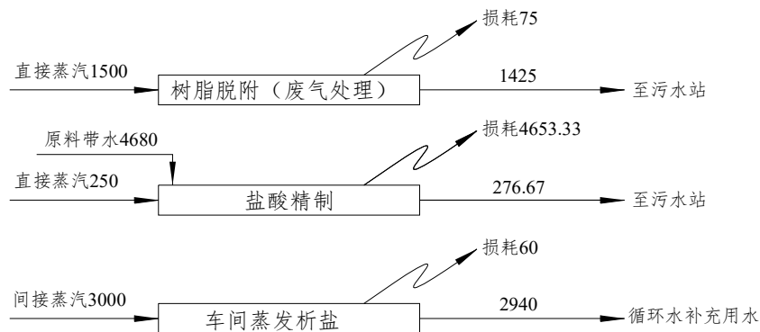
图4.1.4-3 拟建项目蒸汽平衡图 (t/a)
