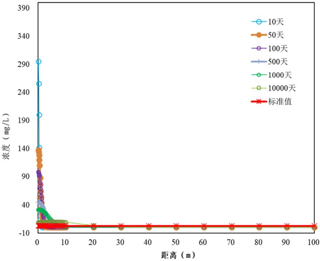
图6.6.3-1 非正常工况下COD Mn 叠加本底浓度变化结果图
