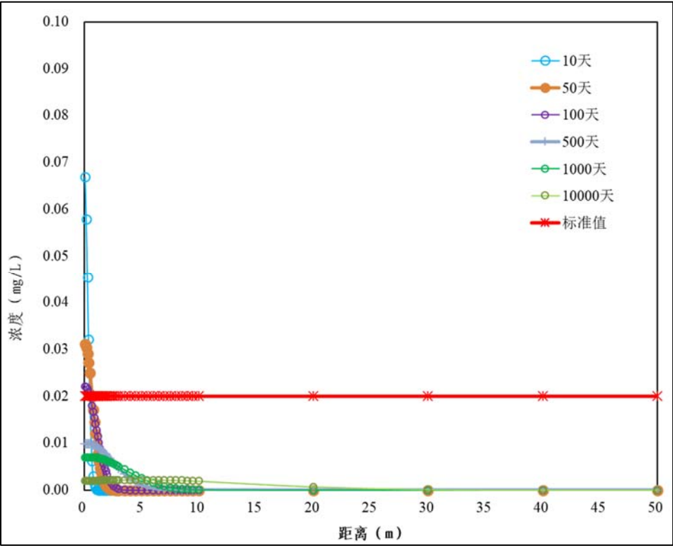
图6.9.3-6 消防废水二氯甲烷下渗浓度变化结果图
