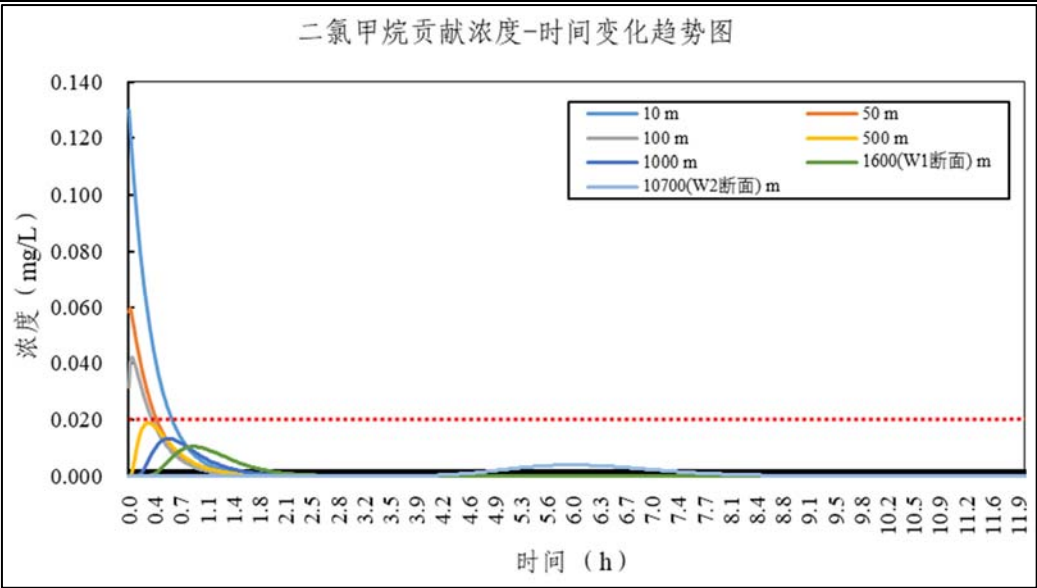
图6.9.3-4 含二氯甲烷消防废水对下游不同距离处二氯甲烷浓度贡献值随时间变化曲线
