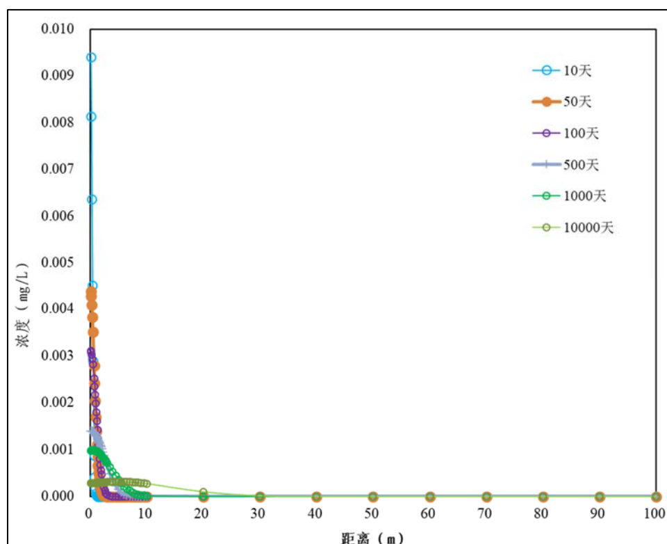
图6.9.3-7 消防废水COD Mn 下渗浓度变化结果图
