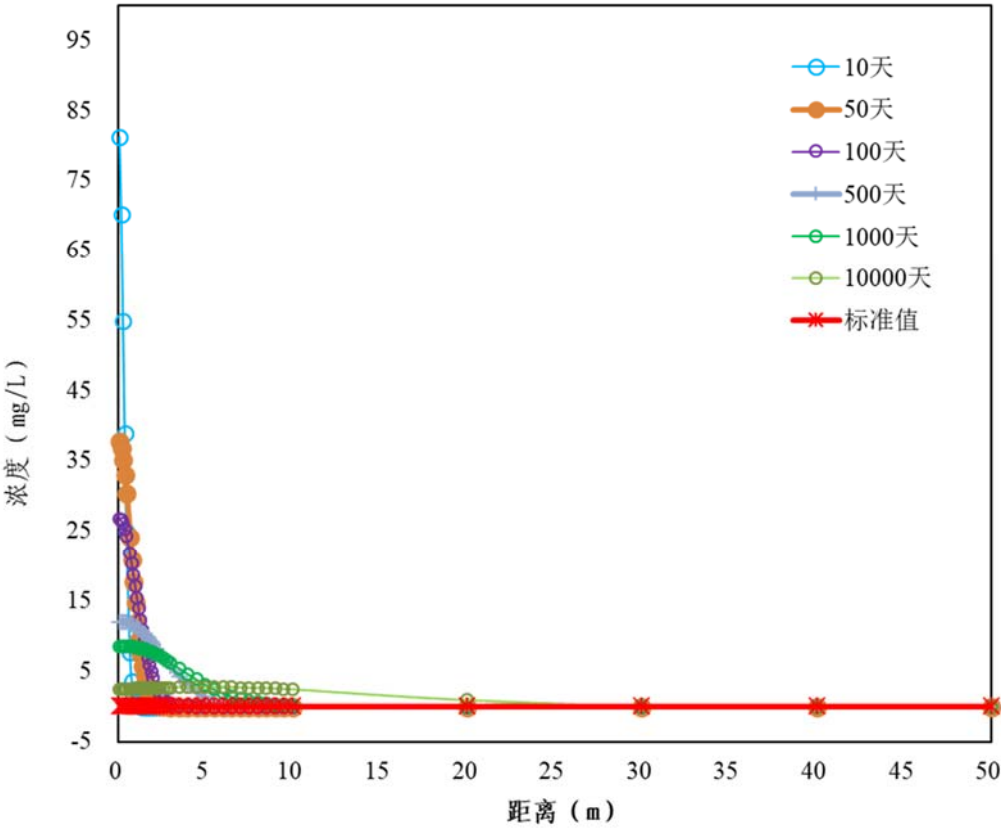
图6.6.3-3 非正常工况下二氯甲烷叠加本底浓度变化结果图
