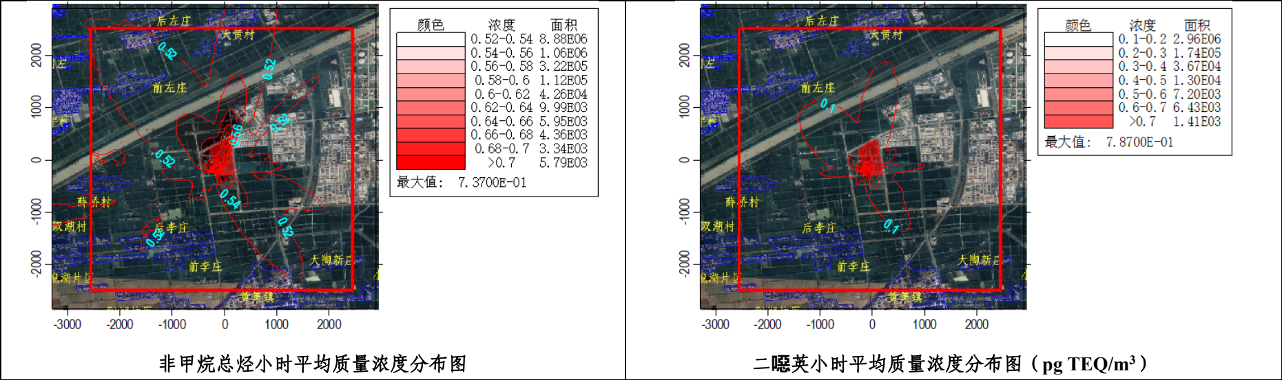
图6.1.4-1 拟建项目质量浓度分布等值线图
