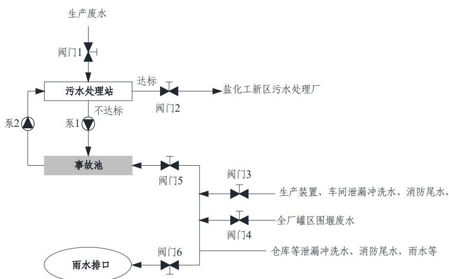
图7.6.1-2 事故废水防范和处理流程示意图
