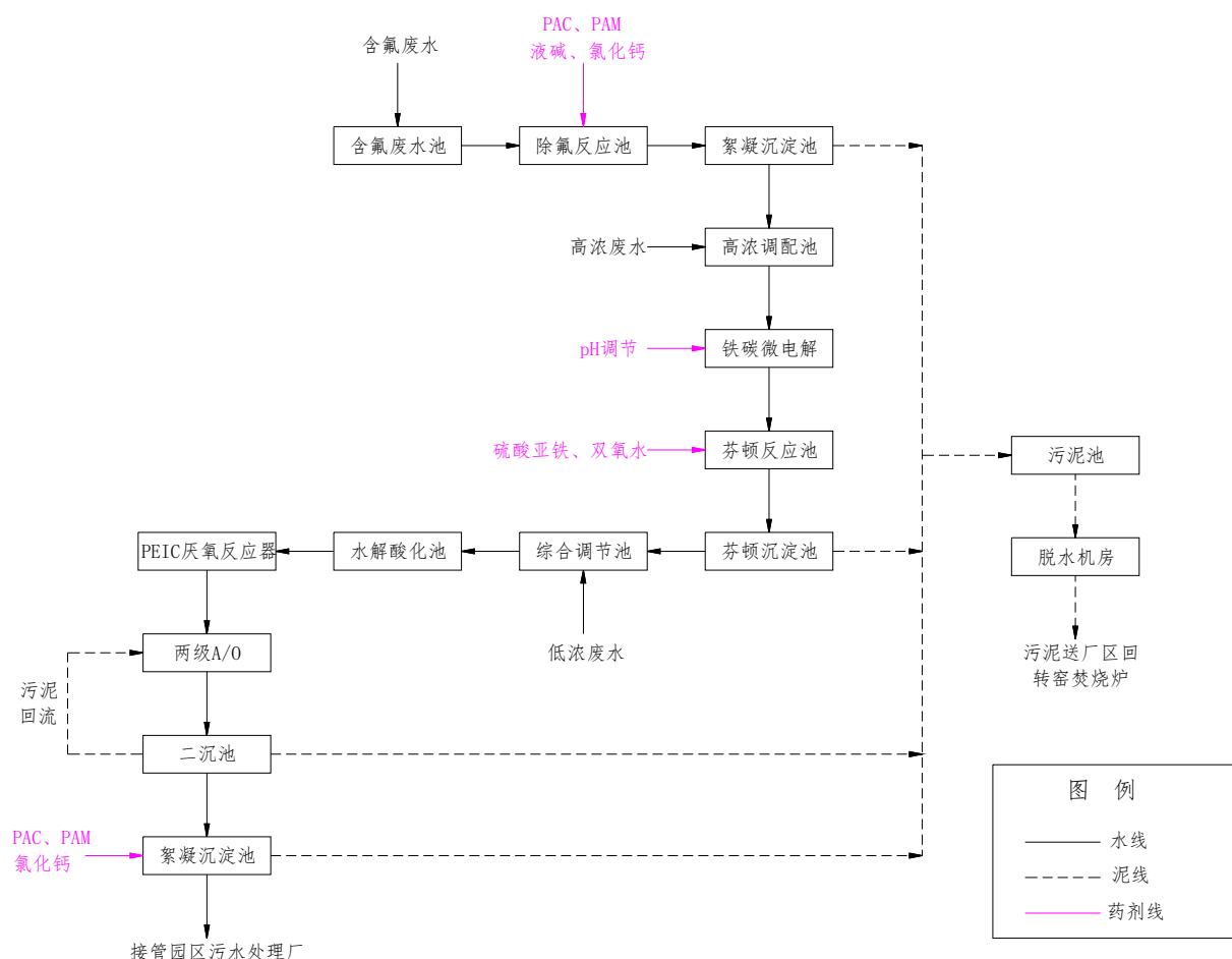
图3.4.2-1 废水处理工艺流程图
