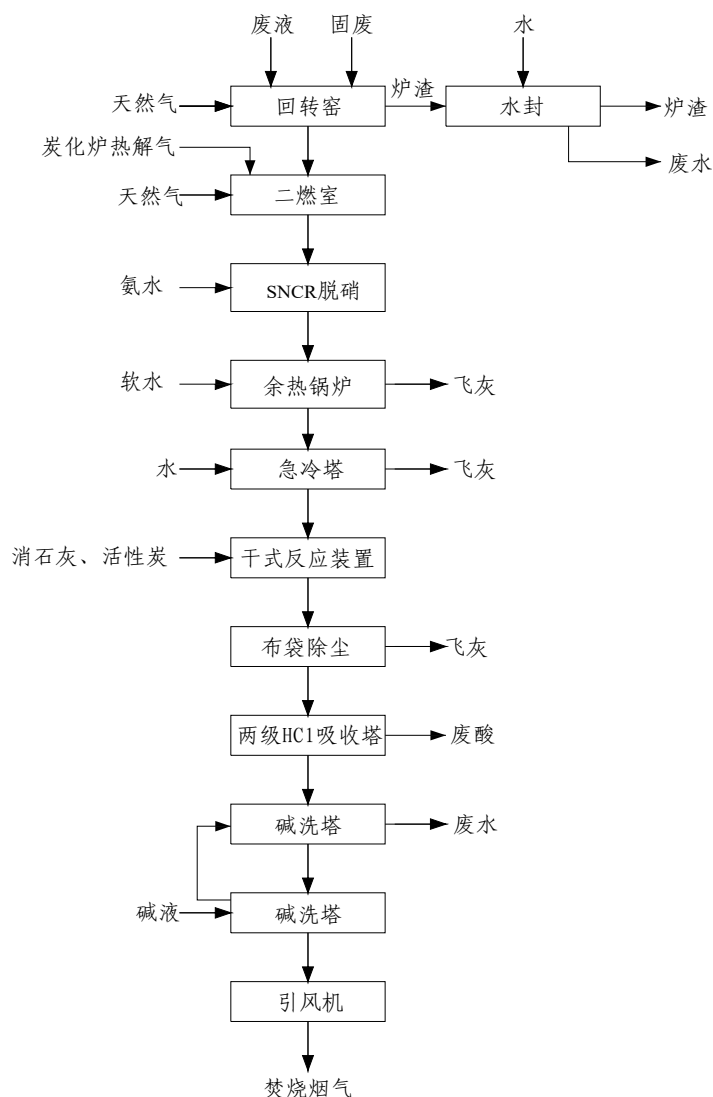
图3.3.2-1 回转窑焚烧炉焚烧工艺流程图
