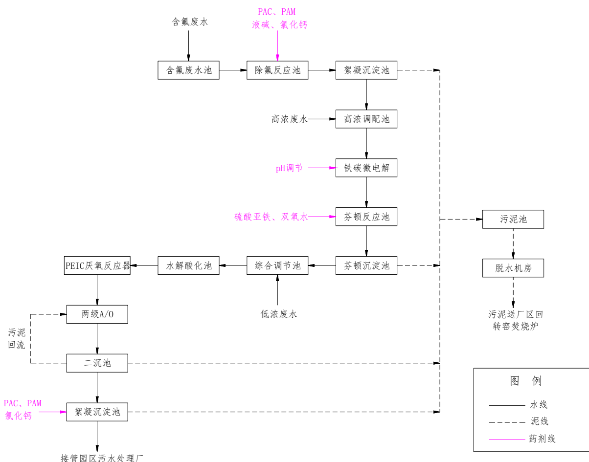
图7.1.1-1 废水处理工艺流程图
