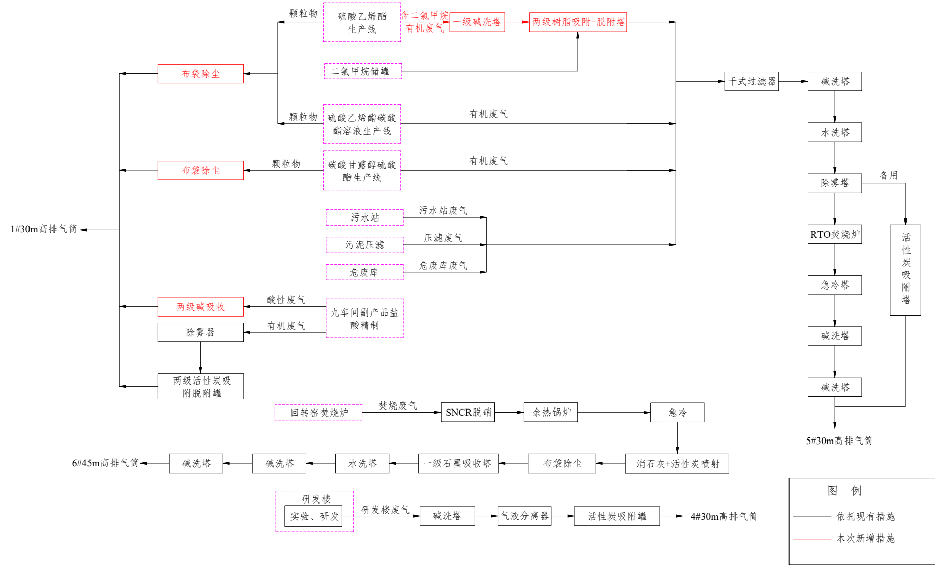
图7.2.1-2 拟建项目废气收集系统和处理工艺流程图
