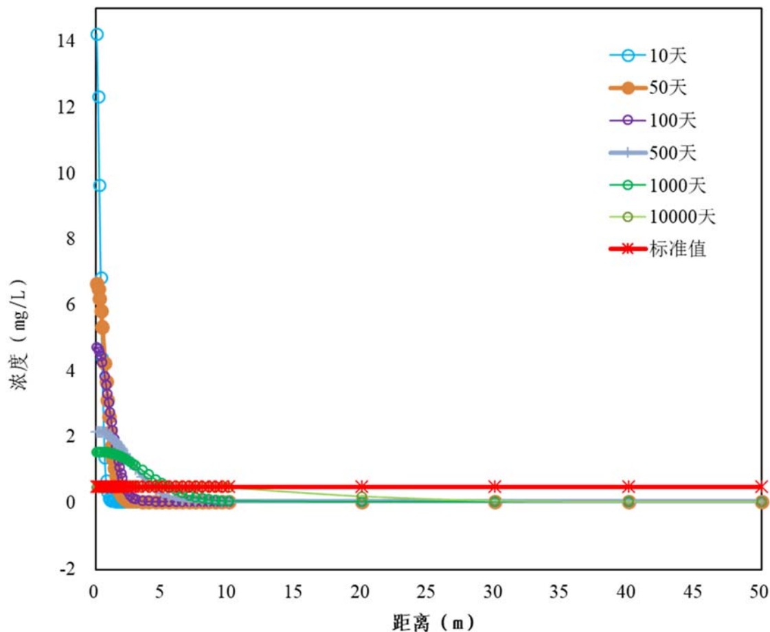
图6.6.3-2 非正常工况下氮氮叠加本底浓度变化结果图
