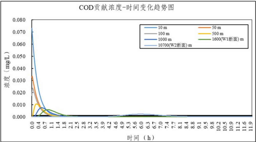
图6.9.3-5 含二氯甲烷消防废水对下游不同距离处COD浓度贡献值随时间变化曲线
