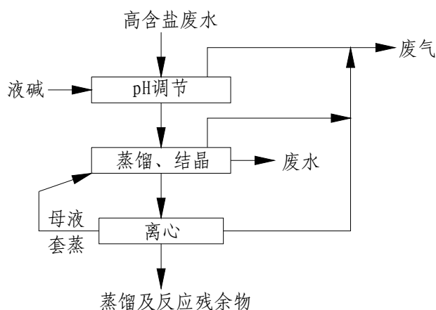
图7.1.2-2 拟建项目高盐废水预处理流程图
