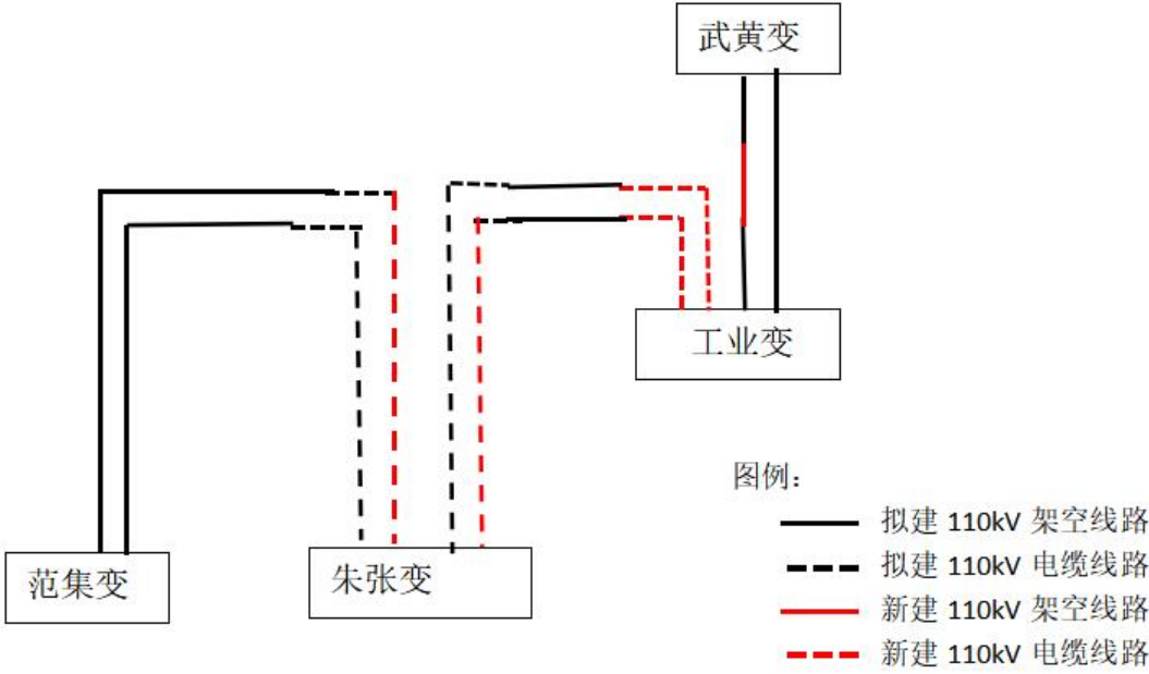
图 2-1 本项目投产前接线示意图
