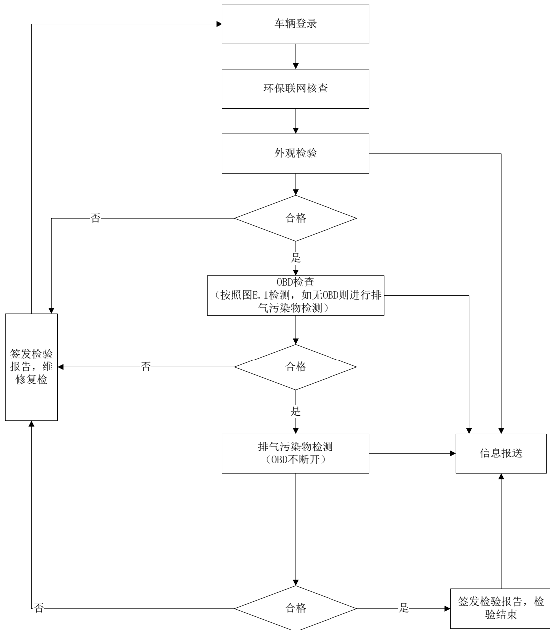
图 3 在用汽车环保检验流程图
